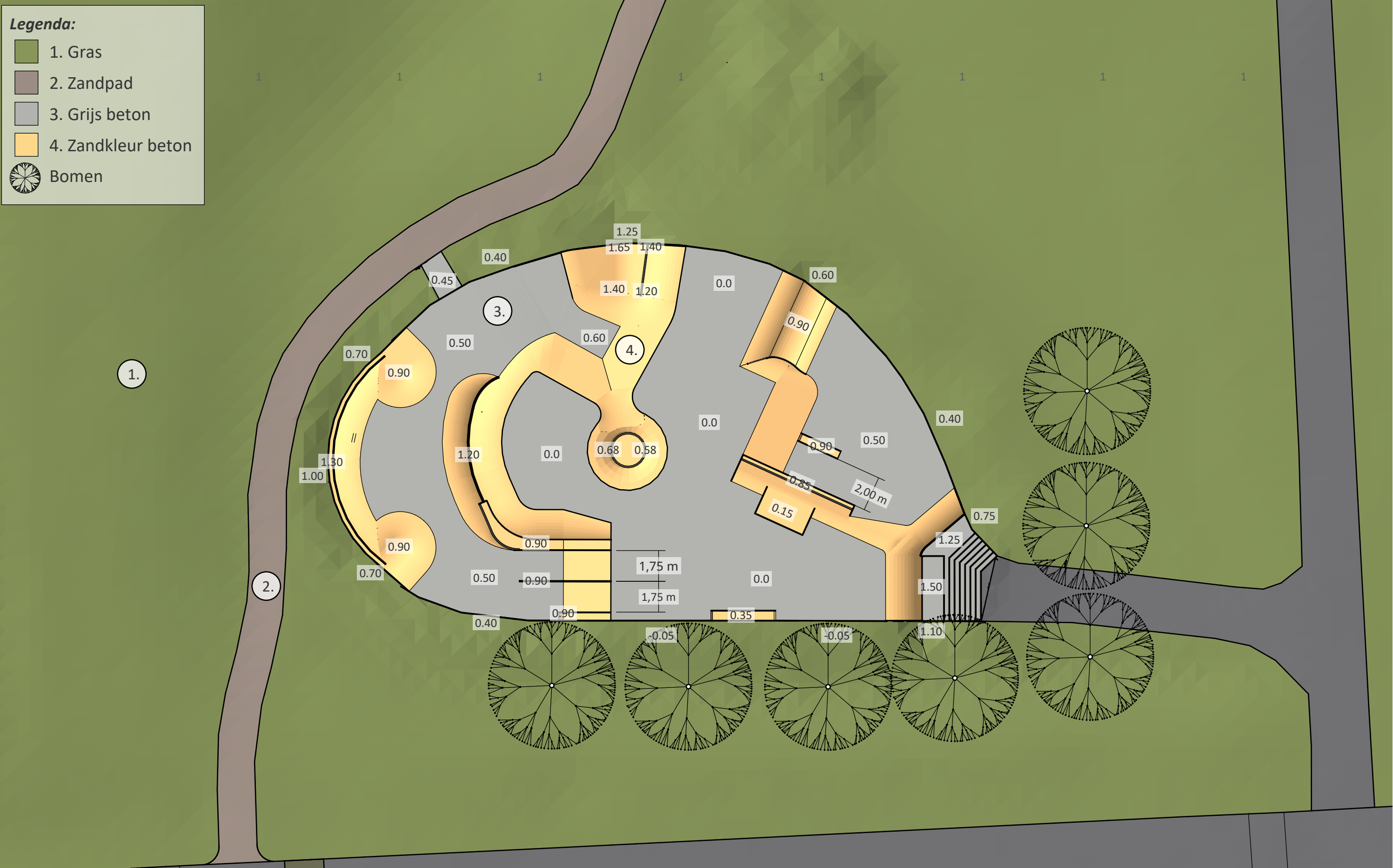
Maten in meter t.o.v. laagste vloer (0.0)
