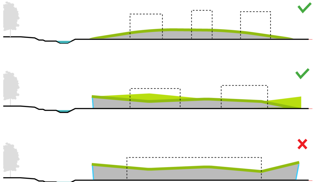
Toelichting bij Eis B.18.5 - Afbeelding aansluiting verhoogde maaiveld op omringend maaiveld
